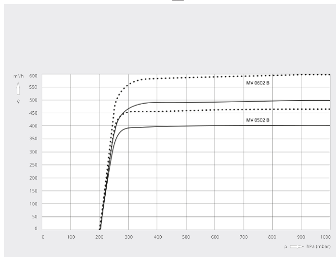
Pumpekapasitet
